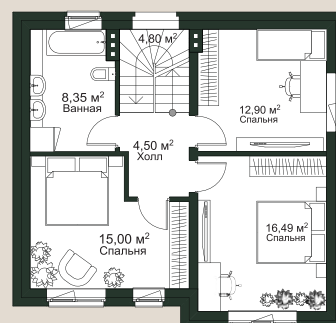
2 этаж
