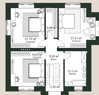
2 этаж
