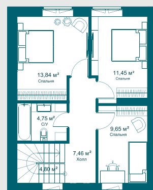
2 этаж
