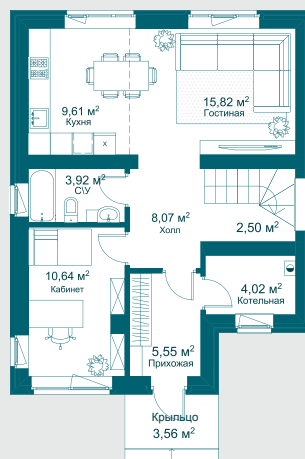
1 этаж
