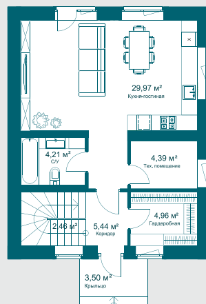
1 этаж
