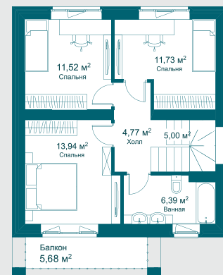
2 этаж
